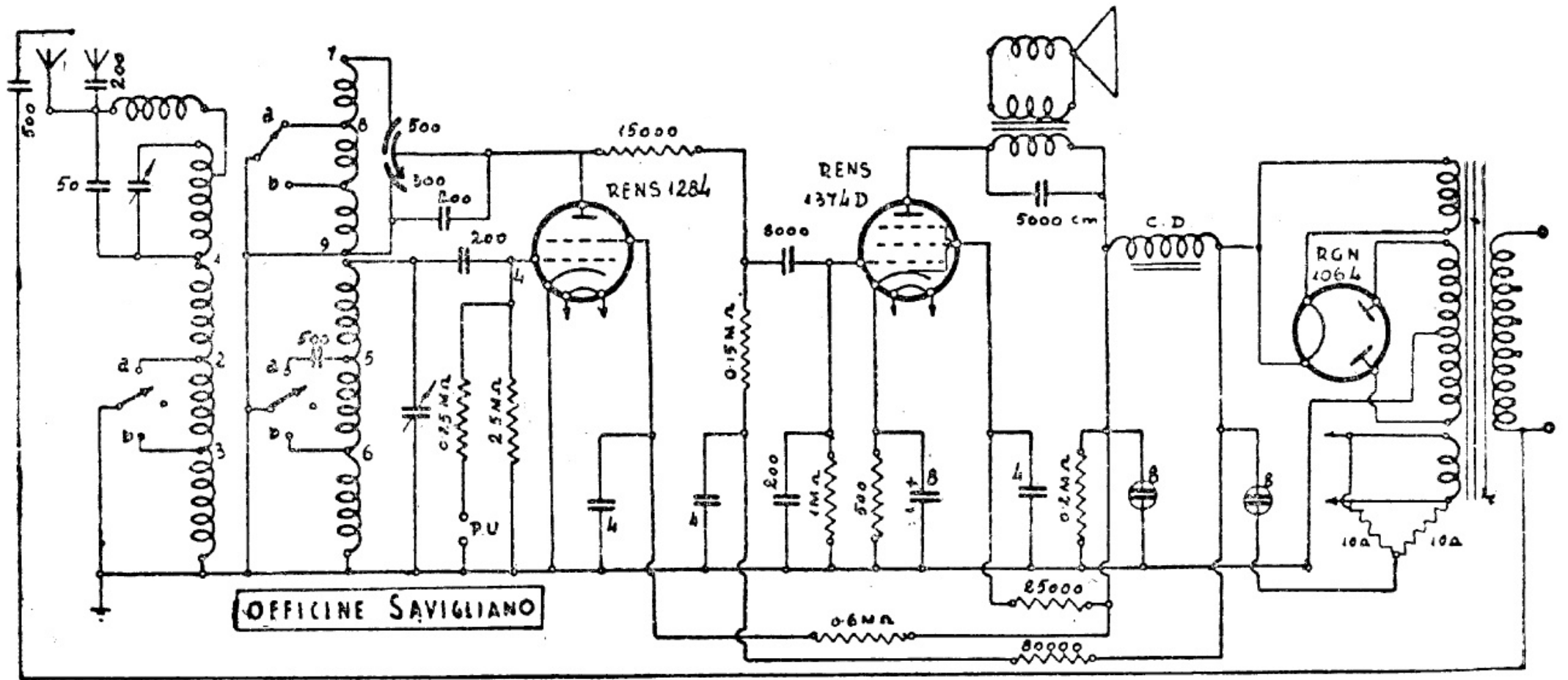
S. A. OFFICINE SAVIGLIANO. — Modello « Tre valvole ». - Produzione 1934.
